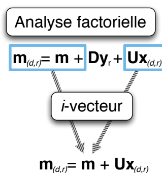
FIGURE 4.1 – Composantes utiles pour l'extraction des i -vecteurs.
